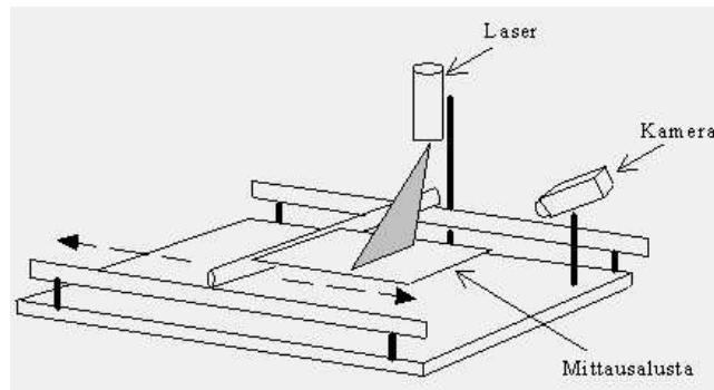
Pöytäskanneri.
