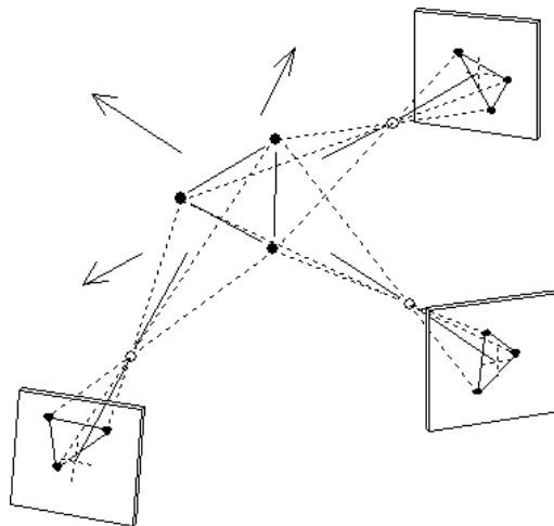
Konvergenttikuvaus.
