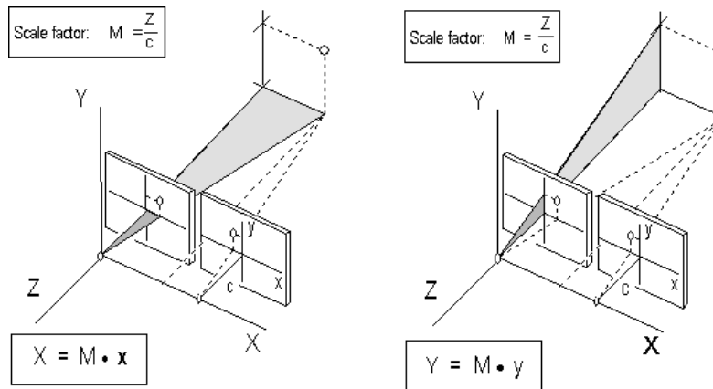
Parallaksikaavat tasokoordinaateille.
